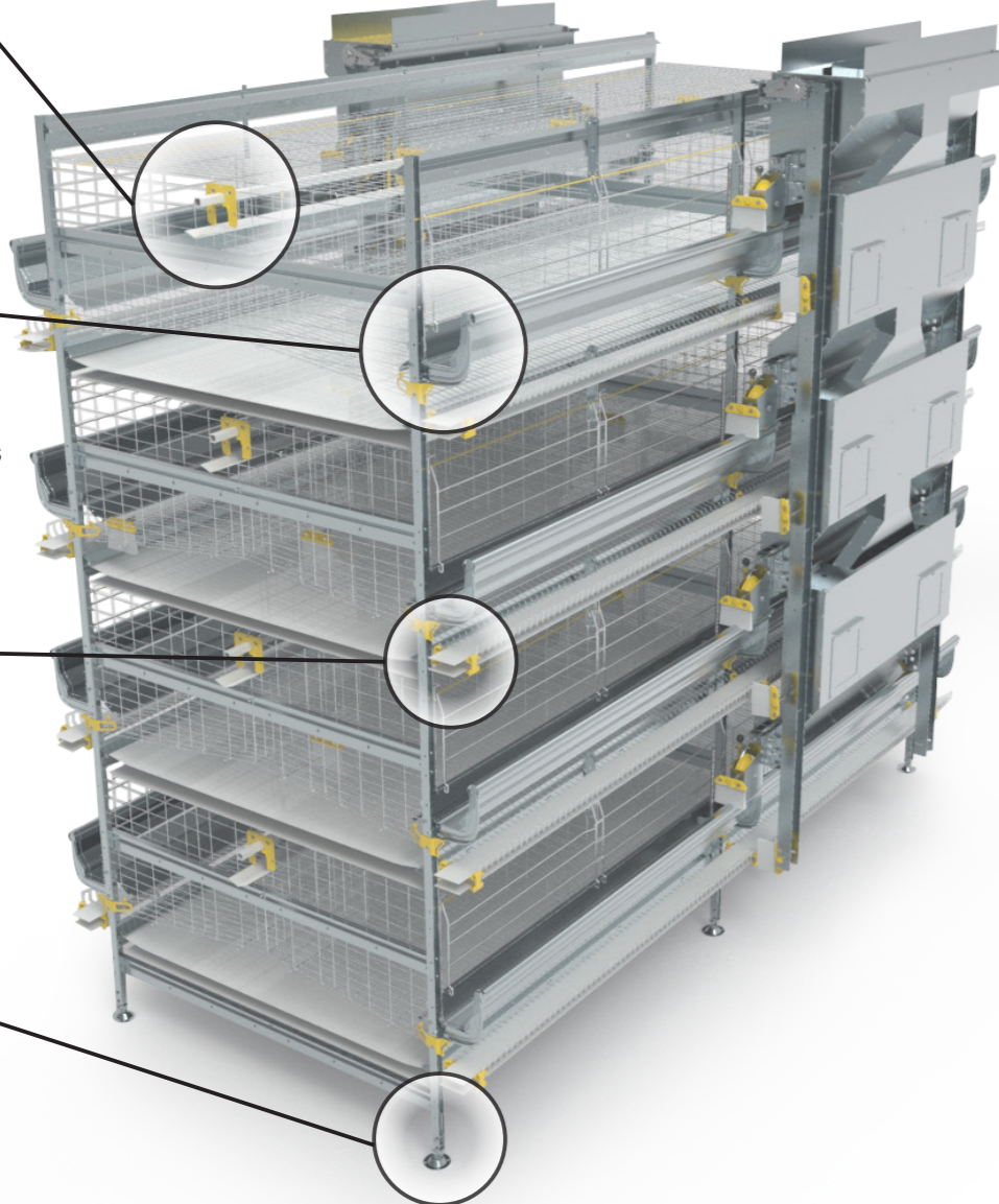
Mangeoires autoportantes
